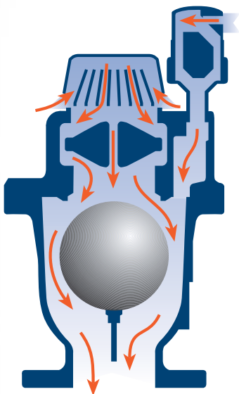
4. עם ירידת מפלס המים במערכת (לעת ניקוז הקו). תת הלחץ שנוצר בשסתום מאפשר למצופף לרדת, לפתוח את הנחיר הקינטי (האוריפיס הגדול), להחזיר את מדף השניקה למצב פתוח (Normally Open) ולהכניס כמות גדולה של אויר לקו.
