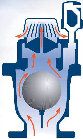
2. כאשר לחץ האויר היפרנציאלי מגיע לרמה קבועה מראש (בד"כ בין 10 ל-35 ס"מ) ייסגר מדף השניקה.
