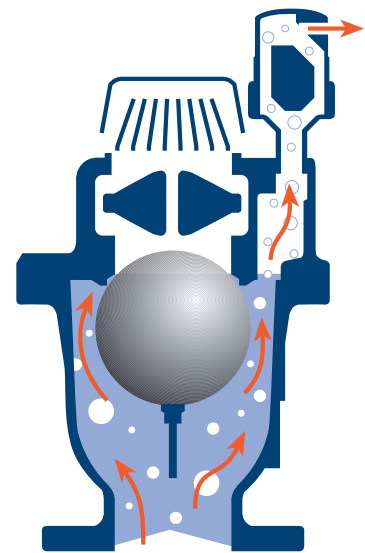
3. אויר ימשיך לצאת דרך הנחיר הקטן של המדף עד ליציאת כל כמות האויר שבשסתום והמים יחדרו ויגיעו למצופף הקינטי ויגרמו לסגירה איטית של המצופף על הנחיר הקינטי. שלב כפול זה של שחרור אויר מבוקר דרך נחיר קטן מאיט את מהירות התנועה של עמוד המים ויוצר כרית אויר זמנית באזור השסתום. פעולות אלו מונעות את סגירת המצופף במהירות ועל ידי כך מונעות את תופעת הטריקה ומפחיתות את הלם המים.
